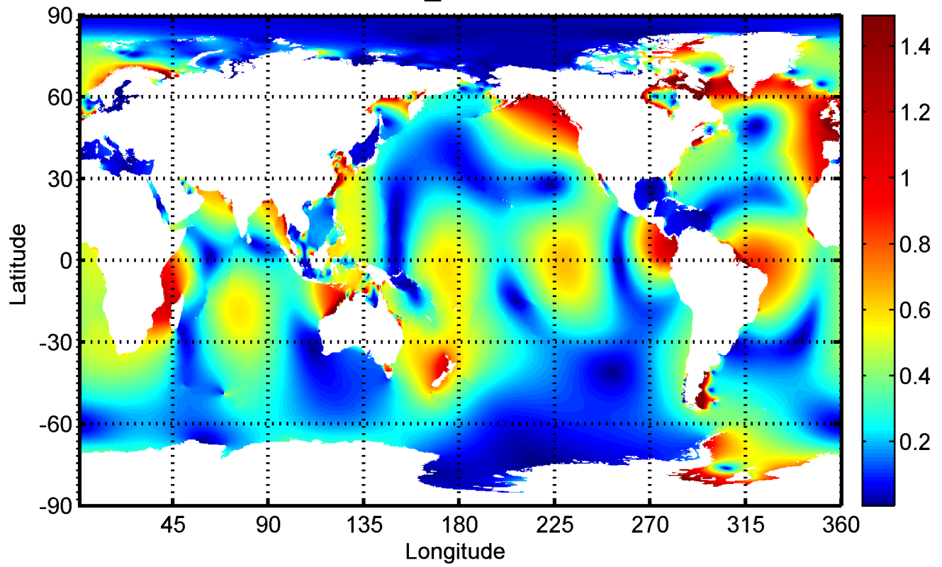
Model_TPXO6.2
